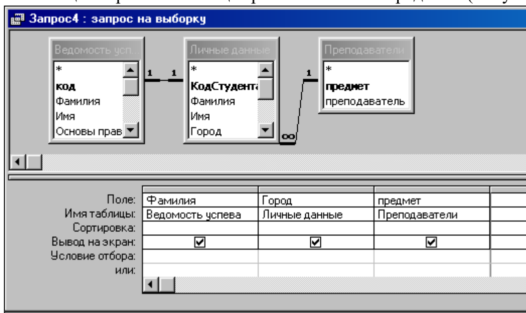
Рисунок 14 – Создание запроса на выборку
