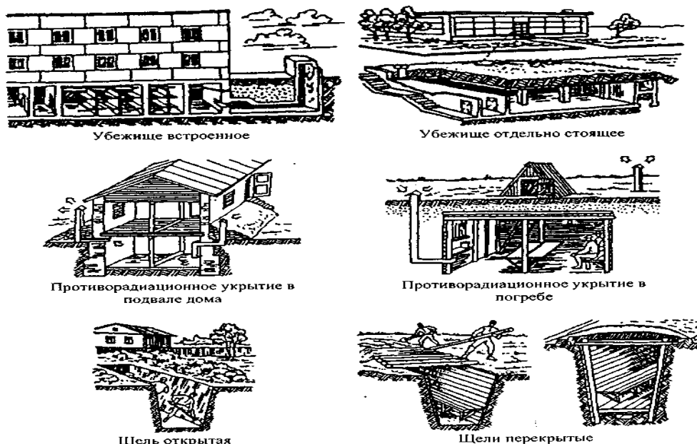
Рис. 2. Защитные сооружения.
