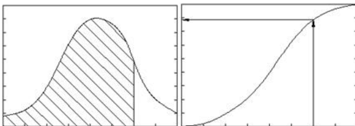
Рис. 2.10. Графическая интерпретация процесса обработки непрерывной случайной величины
