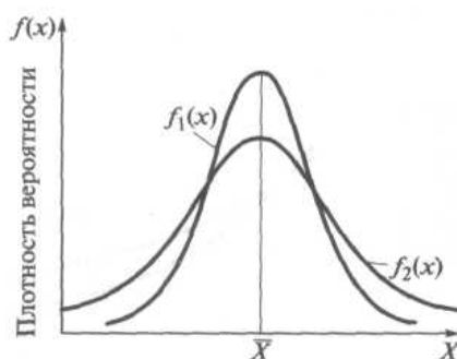
Рис.2.11. Графическая интерпретация нормального распределения
