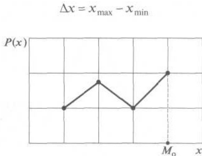
Рис. 2.1 Графическая интерпретация моды дискретной СВ
