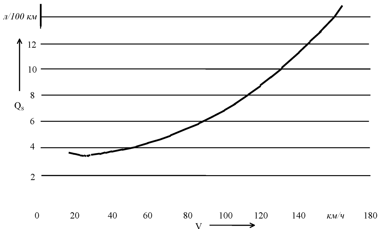
Рис. 4.3. Топливная характеристика установившегося движения
