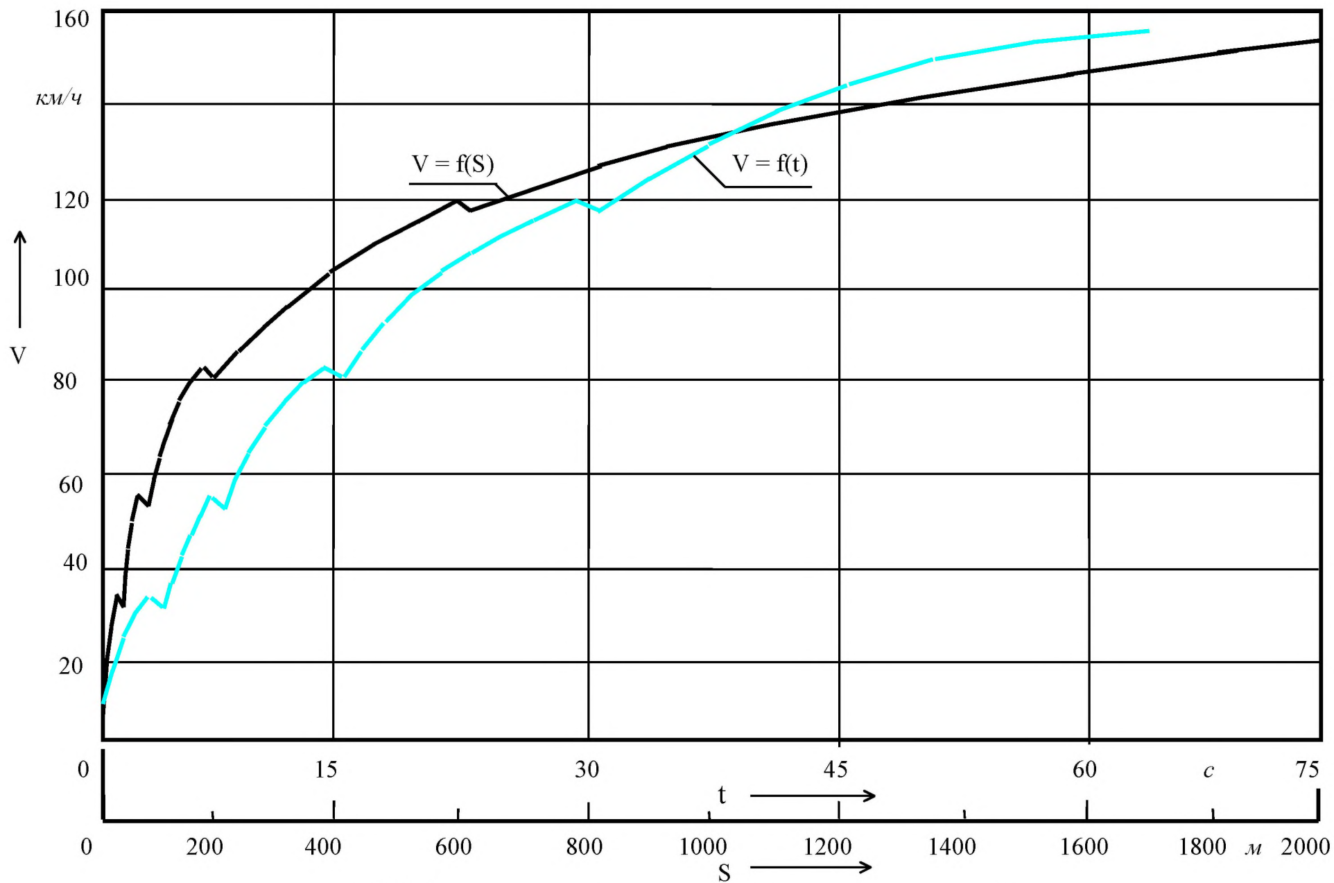
Рис. 3.8. Скоростные характеристики времени и пути разгона автомобиля
