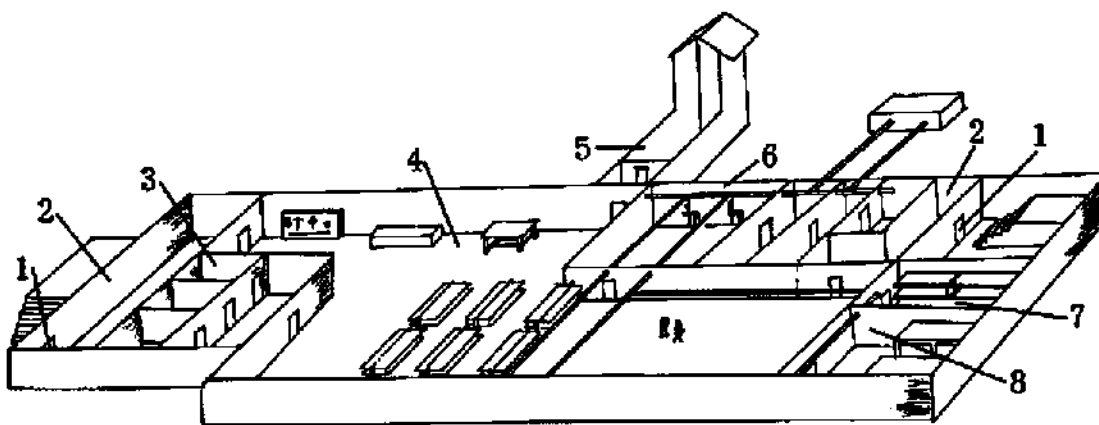
Рис. 4. Планировка убежища: 1 – защитно-герметические двери, 2 – плуксовые камеры, 3 – санитарно-бытовые отсеки, 4 – основное помещение для размещения людей, 5 – галерея и оголовок аварийного выхода, 6 – фильтровентиляционный отсек, 7 – медицинская комната, 8 – кладовая для продуктов
