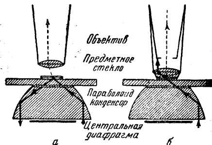
Рис. 20. Ход лучей в микроскопе с темным полем зрения. а — с сухой системой; б — с иммерсионной системой.
