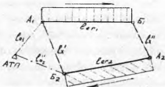
Рисунок 3 – Схема кольцевого маршрута
