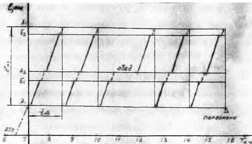
Рисунок 4 – График движения автомобиля на кольцевом маршруте
