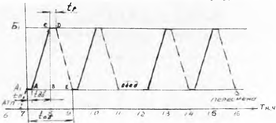
Рисунок 2 – График движения автомобиля на маятниковом маршруте
